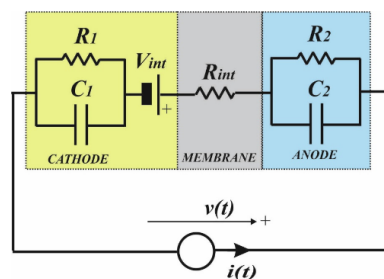
Fig. 1. Equivalent PEM cell circuit [9].
