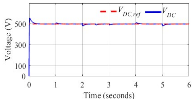
Fig. 19. DC-bus voltage.
