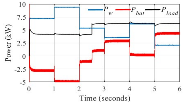
Fig. 23. Power curve.
